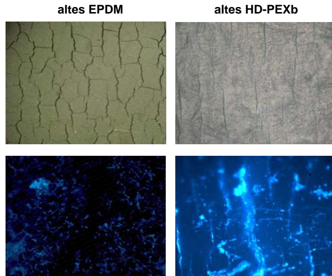
Abbildung 2: oben: Mikroskopische Bilder der Oberfläche von altem EPDM (links) und HD-PEXb (rechts) unten: Fluoreszenzmikroskopische Bilder der besiedelten Oberflächen; Bakterien fluoreszieren als blaue Stäbchen
